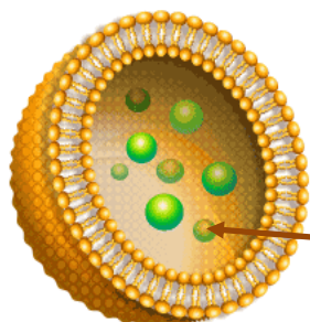
Liposome
